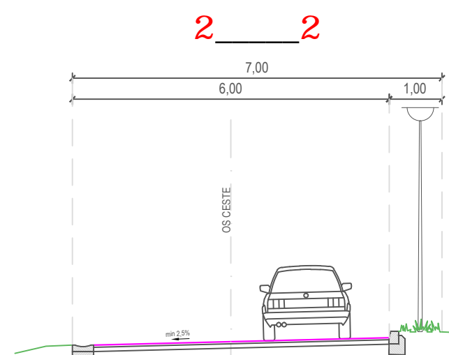
NORMALNI POPREČNI PROFIL
