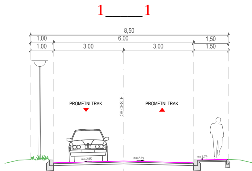
NORMALNI POPREČNI PROFIL
